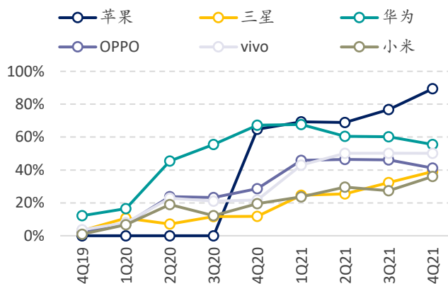
全球智能手机 5G 渗透率按品牌拆分 (4Q19-4Q21)
