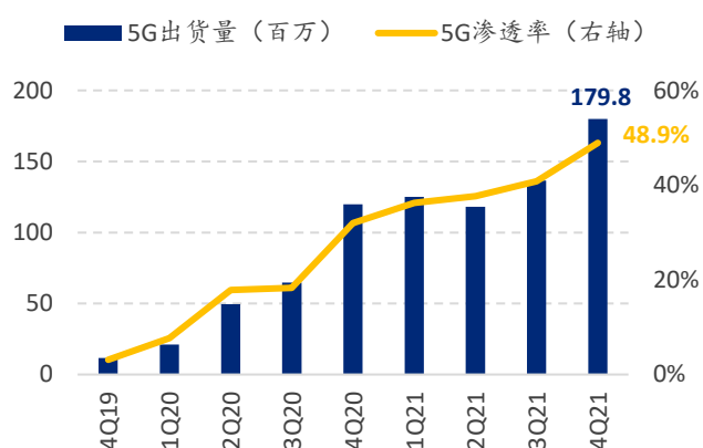
全球 5G 智能手机出货量及 5G 渗透率 (4Q19-4Q21)
